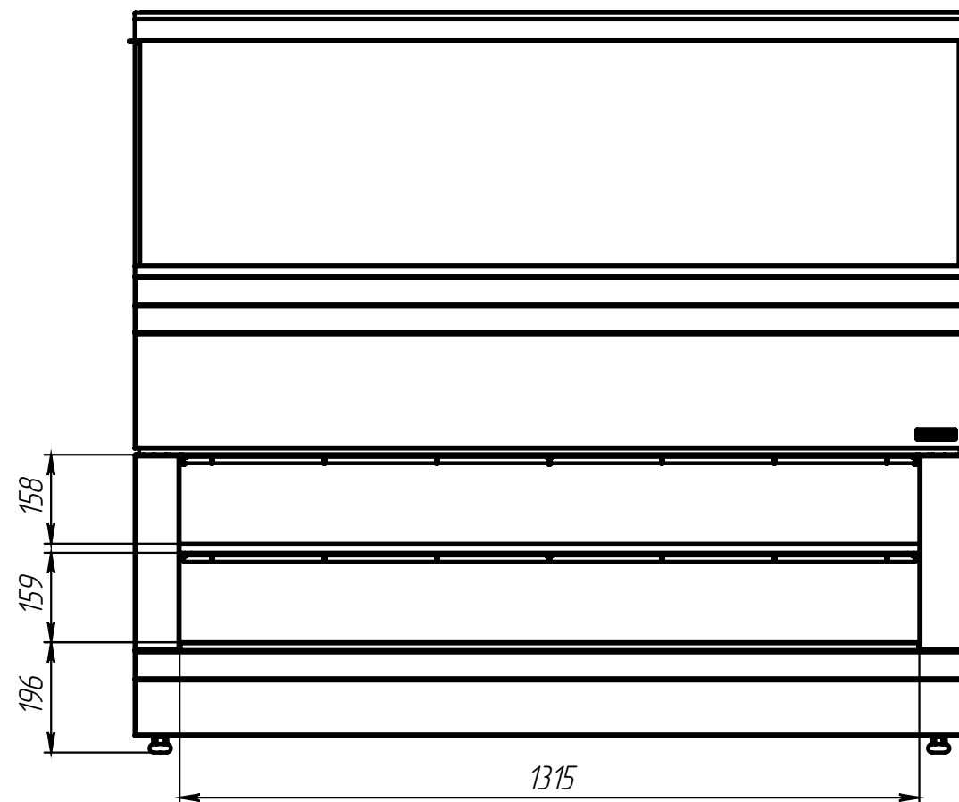
Вариант фасада с нишей
