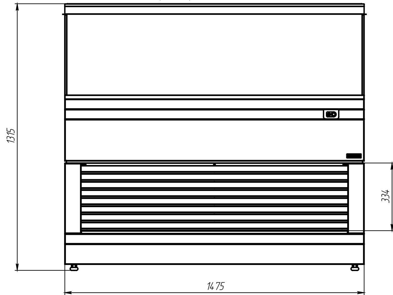
Вариант фасада с жалюзи
